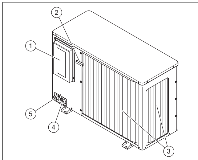
1 Kryt elektrických prípojok 4 Prípojka pre výstup vykurovania, G 1 1/4" 2 Snímač teploty na vstupe vzduchu 5 Prípojka pre spätočku vykurovania, G 1 1/4" 3 Výparník
