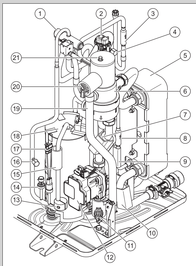
1 4-cestný prepínací ventil 7 Snímač teploty na výstupe, hydraulika 2 Elektronický expanzný ventil 8 Filter 3 Filter 9 Snímač teploty chladiva 4 Údržbová prípojka v oblasti nízkeho tlaku 10 Snímač teploty spätočky, hydraulika 5 Kondenzátor 11 Snímač tlaku hydrauliky 6 Odlučovač chladiva 12 Čerpadlo vykurovania
